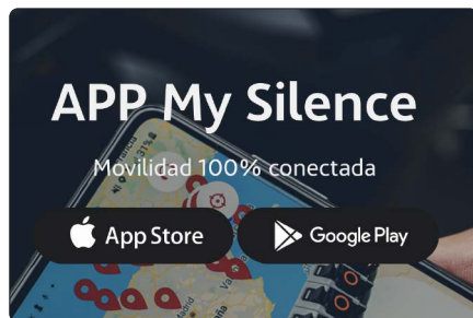
Abb. 116 – APP-Startbildschirm.
